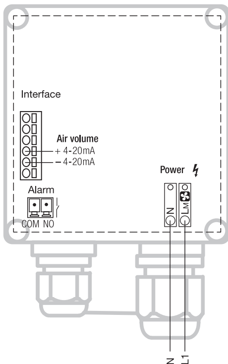
Input 4 – 20 mA
