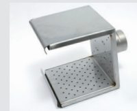
Решетчатый рефлектор 150 x 130 mm Артикул: 107.333
