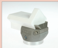
K-30 IA Прямой угловой шов, 30 mm артикул: 145.817
